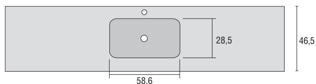
Cod. Vasca B224 cm 58,6 x 28,5 x 13 P
