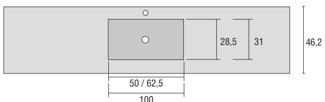
Cod. Vasca B444 cm 50 x 28,5 x 10 P Cod. Vasca B434 cm 62,5 x 28,5 x 11,7 P * Cod. Vasca B448 cm 100 x 31 x 12 P
