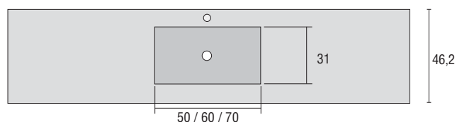
Cod. Vasca B575 cm 50 x 31 x 10,5 P Cod. Vasca B576 cm 60 x 31 x 10,5 P Cod. Vasca B577 cm 70 x 31 x 10,5 P
