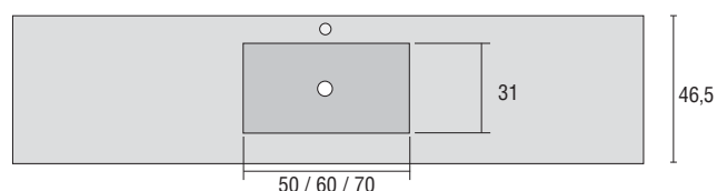
Cod. Vasca B575 cm 50 x 31 x 10,5 P
